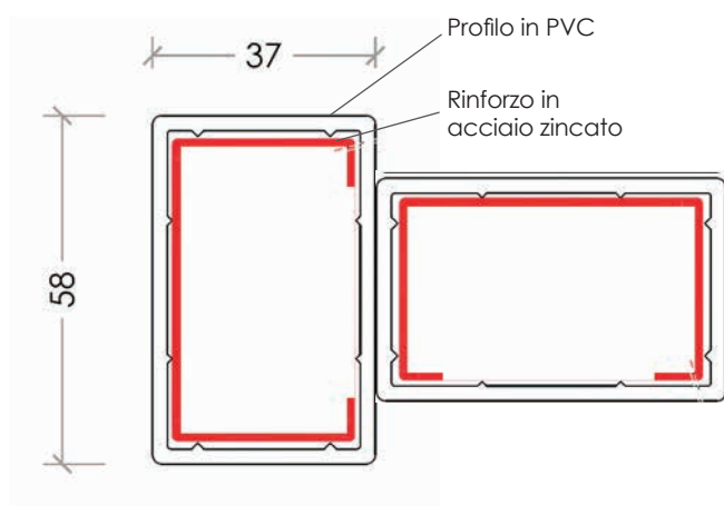
Sezione profilo utilizzato
